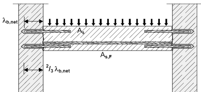
Abbildung A3: Endverankerung von Platten oder Balken, bemessen als Einfeldträger
