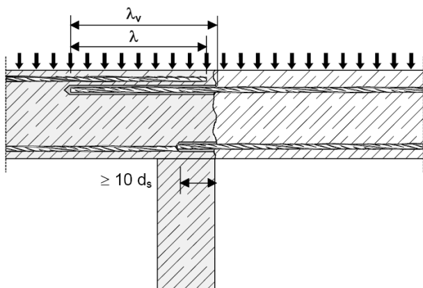
Abbildung A1: Übergreifungsstoß in Platten und Balken
